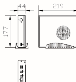
外形図
